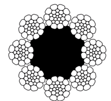
8xK26WS - FC
