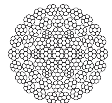
57xK7
