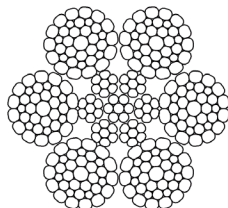
6xK36WS - IWRC
