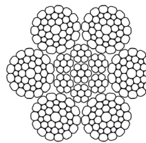
6xK36WS - PWRC
